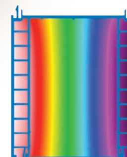
Die Thermographie stellt die Wärmeverteilung in einem 100 mm-StyroClick-Verlängerungsprofil dar.
