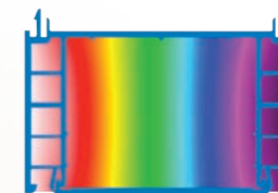
Thermographischer Querschnitt eines 50 mm StyroClick-Verlängerungsprofils.
